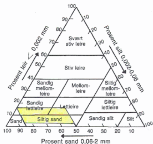
Figur: Teksturtrekant med anbefalt tekstur for anleggsjord markert med gult felt. Trond Knapp Haraldsen, Bioforsk
